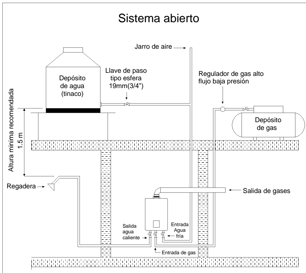
Sistema abierto (por medio de tinaco) para alimentación al calentador. Se debe instalar en la salida de agua caliente un jarro de aire.
