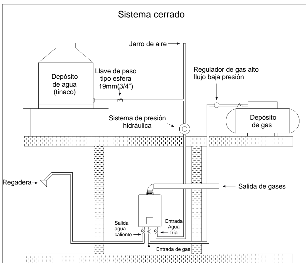
Sistema cerrado para alimentación de agua al calentador. Se debe instalar en la salida de agua caliente una válvula de alivio calibrada a lo que especifique el fabricante del calentador.
