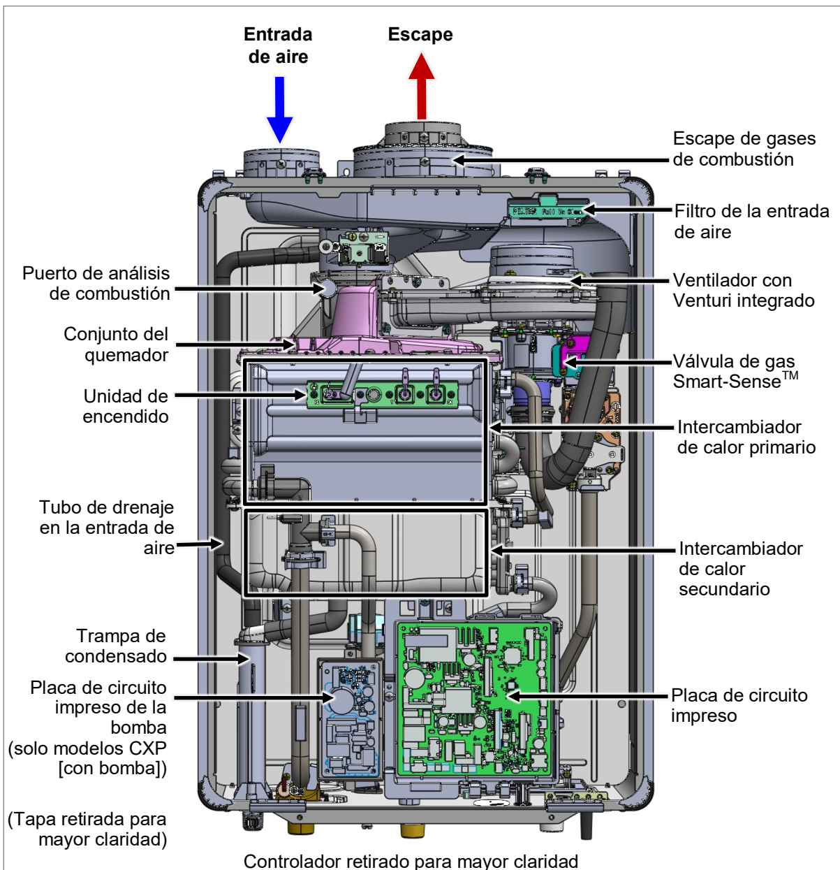
Figura 1: Componentes
