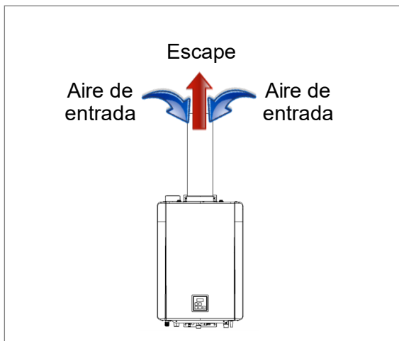
Figura 10: Tubo concéntrico
