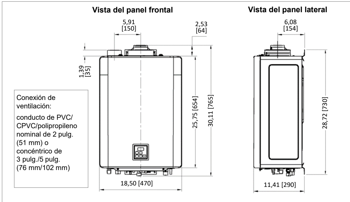
Figura 2: Dimensiones
