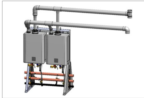
Figura 36: Ejemplo de configuración en línea independiente
