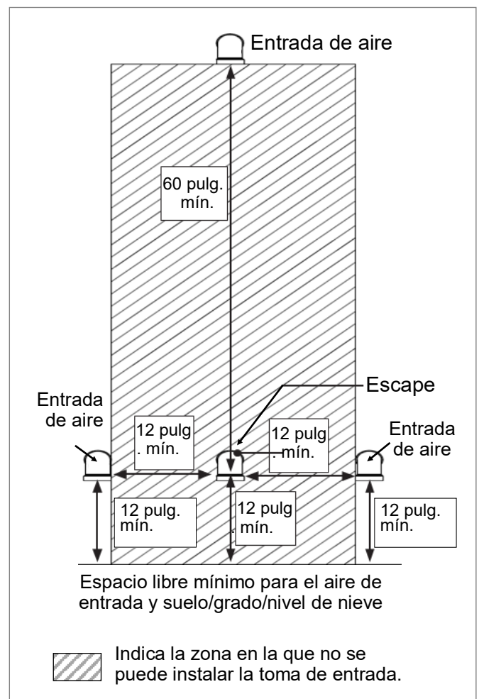
Figura 21: Ventilación horizontal y tuberías de entrada de aire
