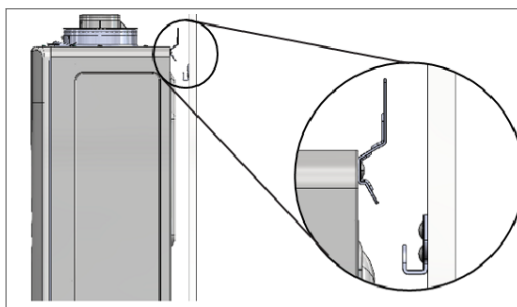
Figura 6: Montaje del soporte superior
