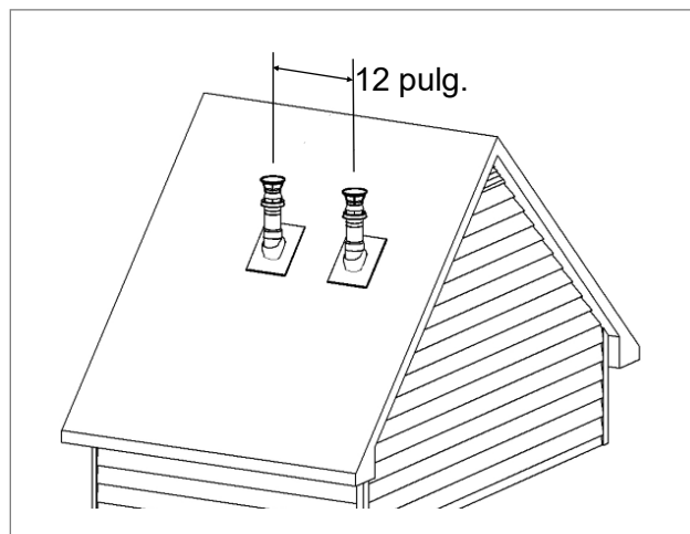
Figura 13: Entre terminales al mismo nivel
