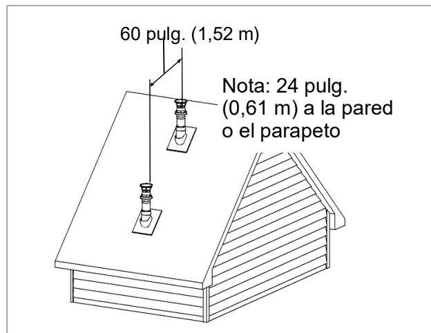
Figura 12: Entre terminales de distintos niveles
