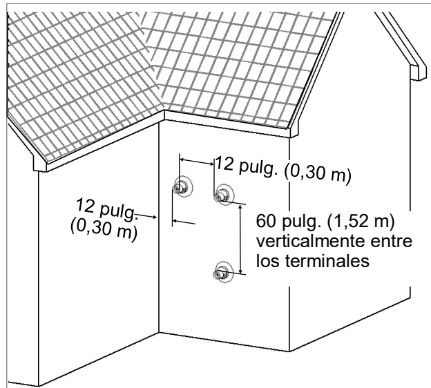
Figura 11: Espacios libres de la terminación del tubo concéntrico
