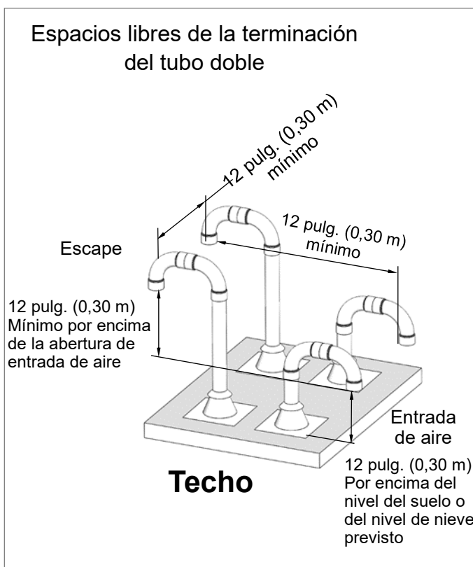
Figura 20: Terminación vertical de tubo doble de varios calentadores de agua
