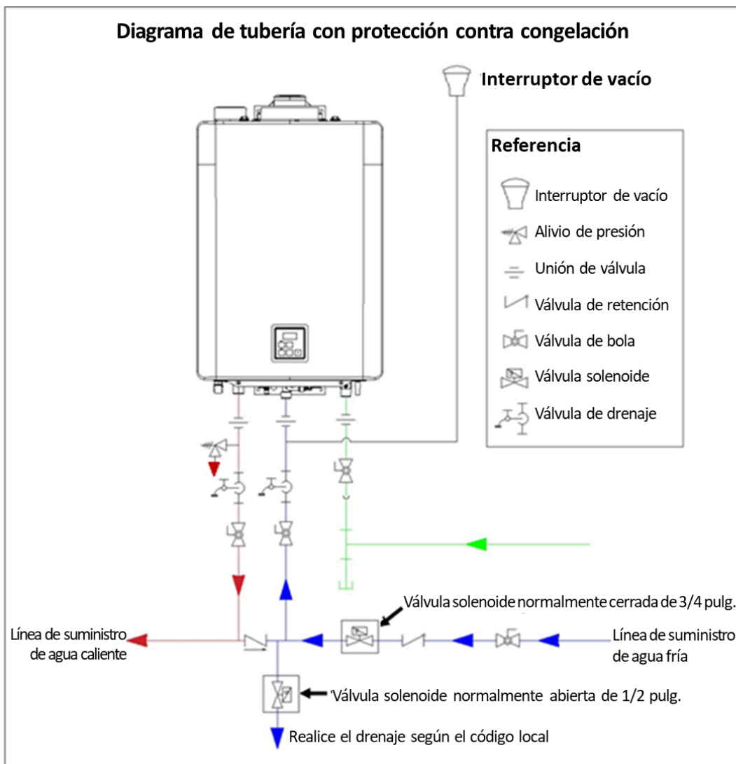
Figura 4: Diagrama de tubería con protección contra congelación
