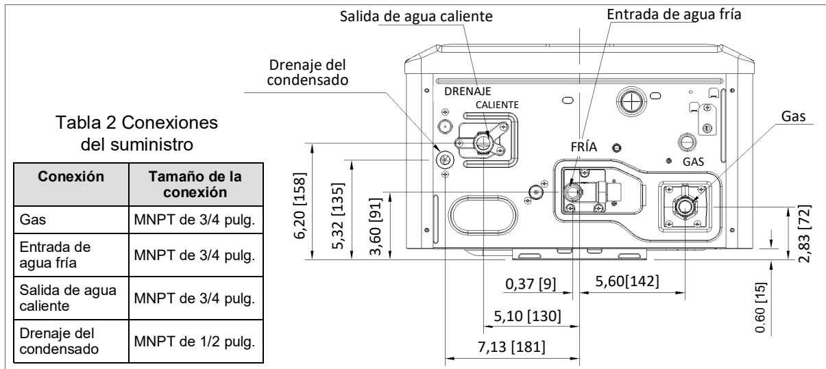
Figura 3: Conexiones del suministro
